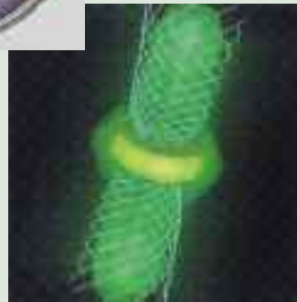
宇宙ジェットのシミュレーション
