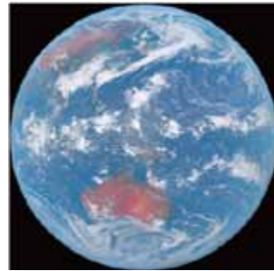
CEReSで処理したひまわり8号の高解像度カラー画像
