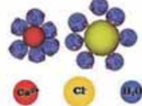
0.5nmのスリット状カーボンナノ細孔に閉じ込められたCaCl 2 溶液の特異的水和構造
