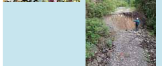
2016年熊本地震の地表地震断層
